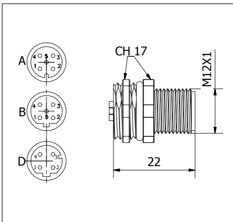
M12 Maschio/Male/Stecker
