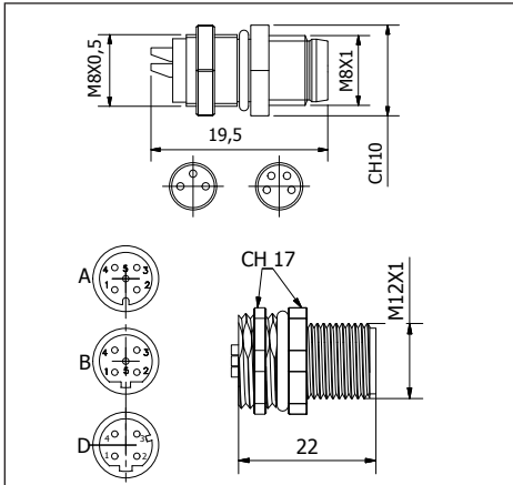
M12 Maschio/Male/Stecker
